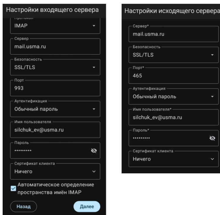
Рисунок 5 – Дополнительные настройки почтового приложения на мобильном устройстве
